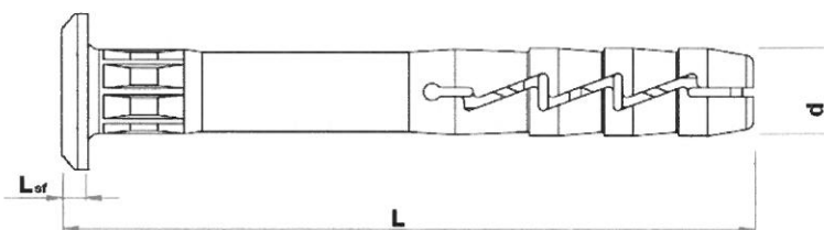
FX-..K.. sleeve
