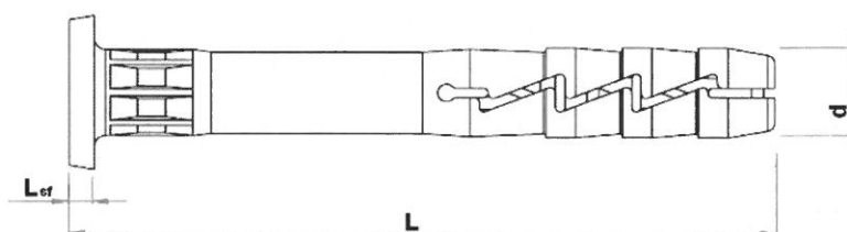
FX-..C.. sleeve
